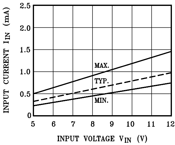
I_{IN} - V_{IN}
