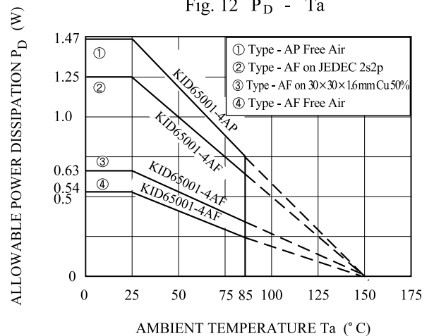
Fig. 12 P_D - T_a
