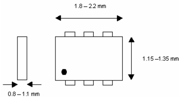
SOT-363
