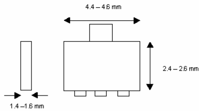
SOT- 89
