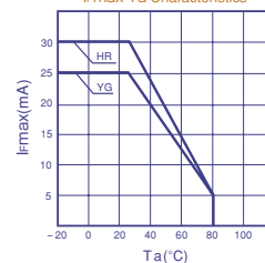
I Fmax -T a 特性 I Fmax -T a Characteristics
