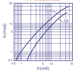
I v -I F 特性 I v -I F Characteristics
