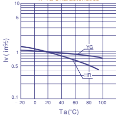
I v -T a 特性 I v -T a Characteristics
