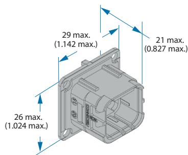
RECEPTACLE
