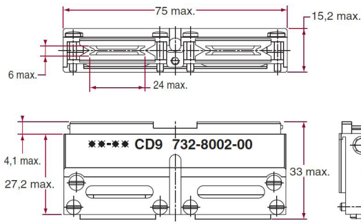
732-8002-00 4 Module Version
