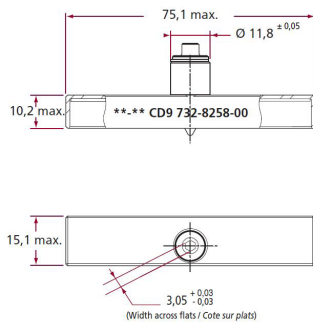
732-8258-00
