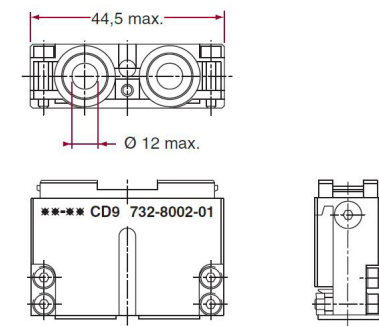
732-8002-01 2 Module Version
