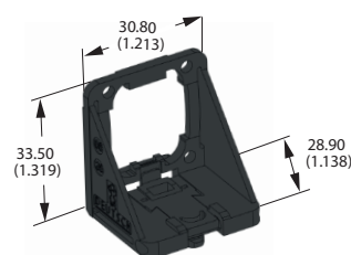
787-8014-00
