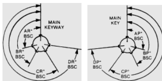
Receptacles
