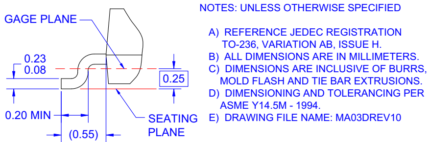
DETAIL A SCALE: 2X
